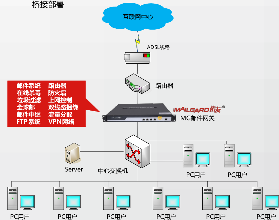
工控版邮件网关（邮件+防火墙二合一） 桥接部署
