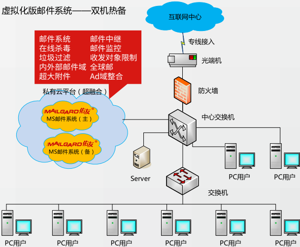
虚拟化版邮件系统——双机热备
